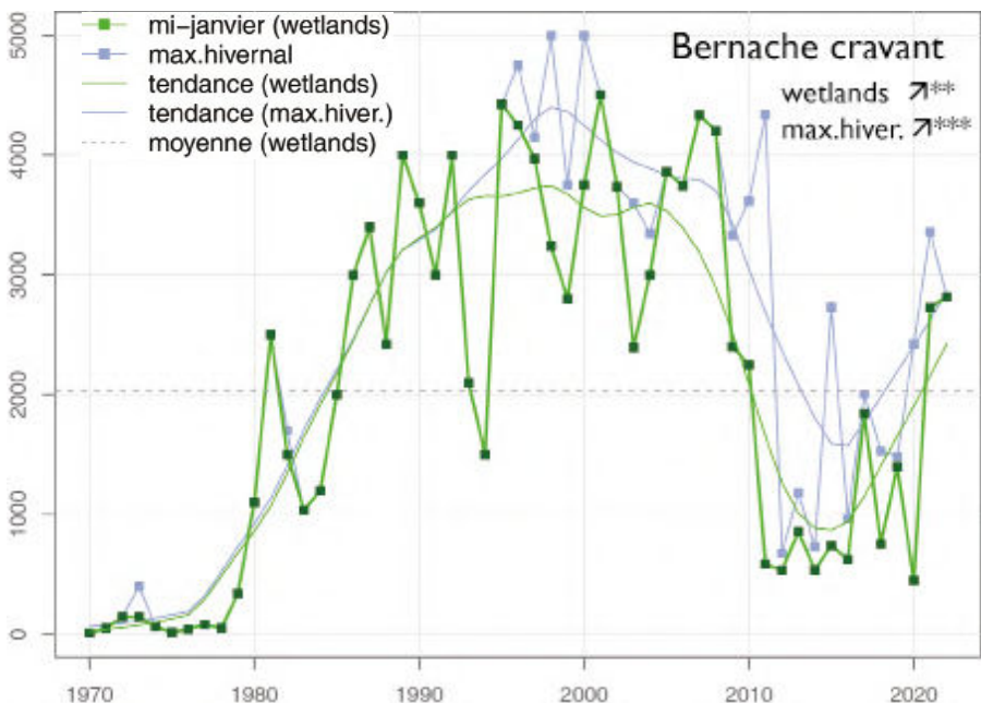
Figures 5 : exemples des principaux patrons d'évolution (augmentation, stabilité, diminution) des effectifs observés sur la période 1970-2022 dans la RNN de la baie de Saint-Brieuc.
