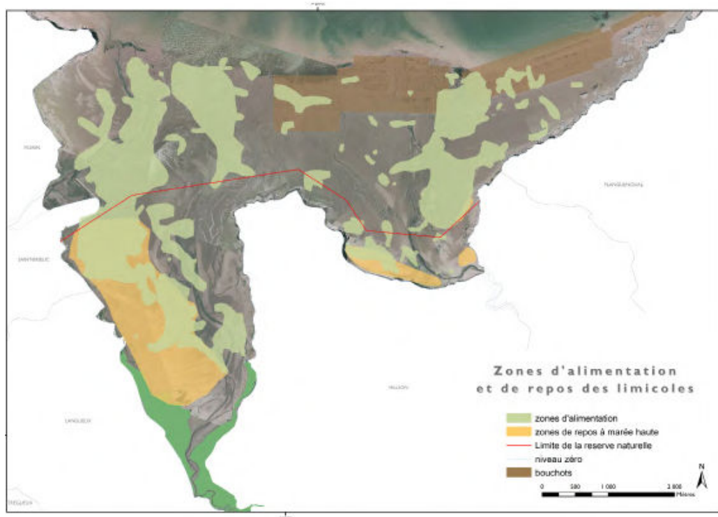
Figure 6 : carte des principaux reposoirs et zones d'alimentation des limicoles en fond de baie de Saint-Brieuc sur le secteur de la Réserve Naturelle.
