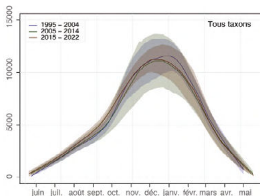
Figure 4 : phénologie des effectifs totaux d'oiseaux hivernants, et des communautés d'anatidés et limicoles présents en fond de baie dans la RNN de la baie de Saint-Brieuc. Trois périodes sont différenciées : 1995-2004, 2005-2014, 2015-2022.
